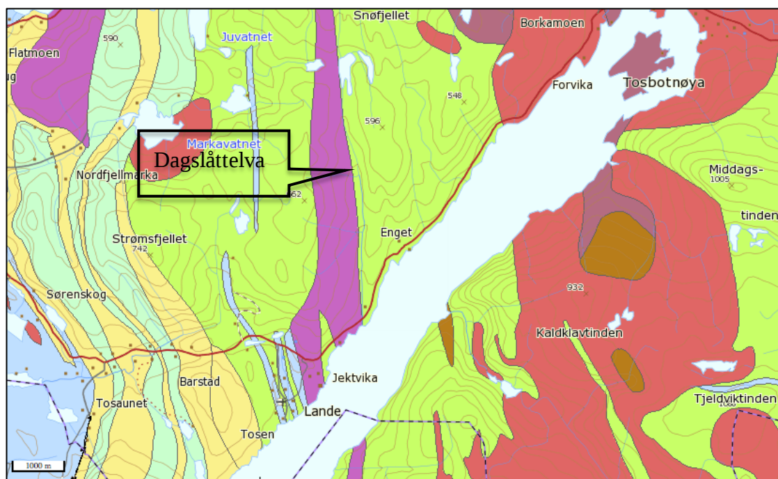
Figur 9. Berggrunnskart over området rundt Dagslåtrelva. Den grønne fargen på østsiden av elva indikerer en samlegruppe av glimmerskifer, gneis, amfibolitt og metasandstein. lilla farge på vestsiden indikerer dioritt og monzonitt. Kilde: Norges geologiske undersøkelse.
